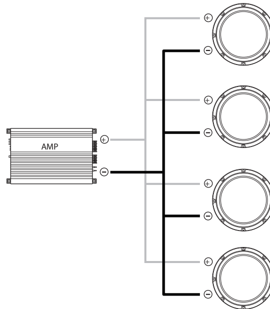
Four Speakers wired in parallel (Cuatro Oradores alambraron en la paralela, Quatre Haut-parleurs ont télégraphié dans l'analogie, Vier Sprecher haben parallel verdrahtet):
